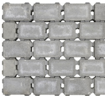
Ökorasenverbundstein anthrazit 24 x 16 x 8 cm Verlegung im Halbsteinverband
